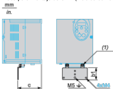
(1) 2 tornillos M5
